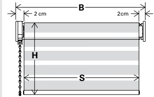
Doppelrollo Seitenzug
